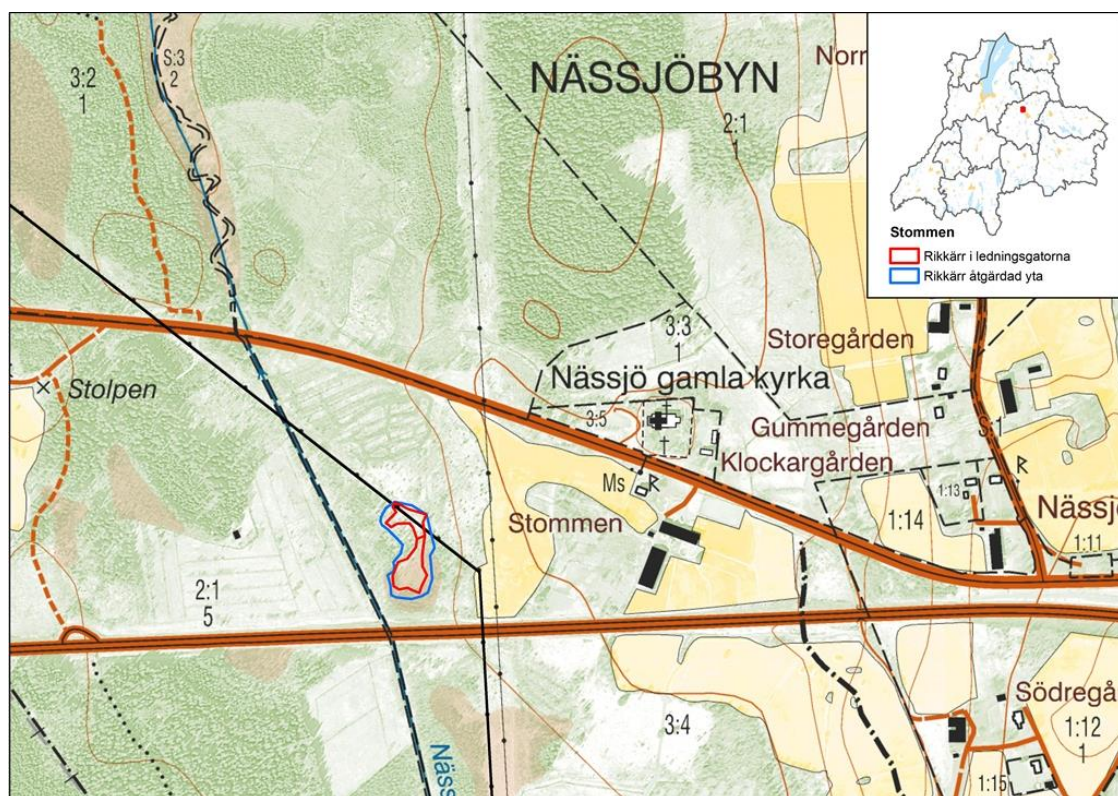
Figur 5. Kartbild över rikkärrsytor (rödmarkerade) och restaureringsytan (blåmarkerad).
