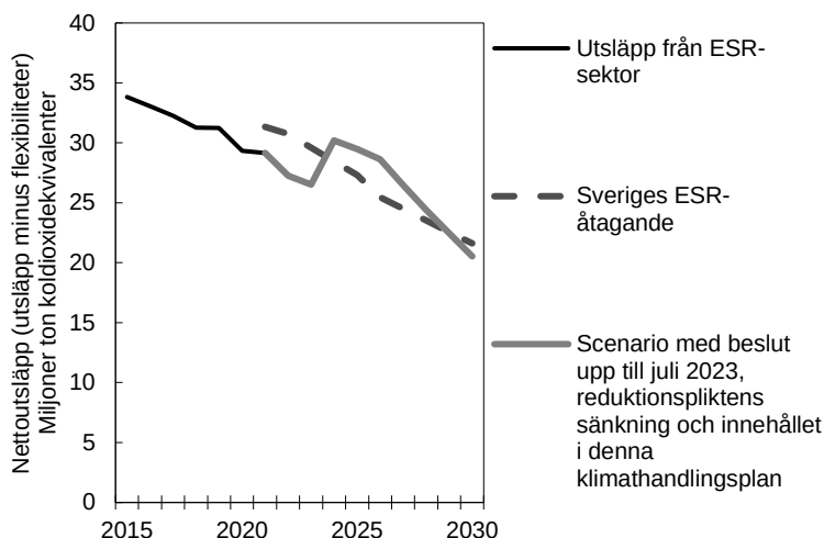
Figur 14.2 Scenario över utsläpp minus flexibiliteter för Sveriges EU-åtagande inom ESR
