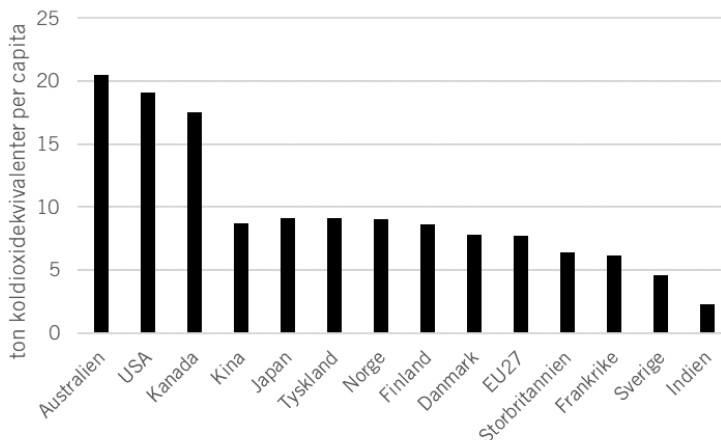
Figur 3.5 Per capita territoriella utsläpp 2020 alternativt 2021 för ett antal utvalda länder
