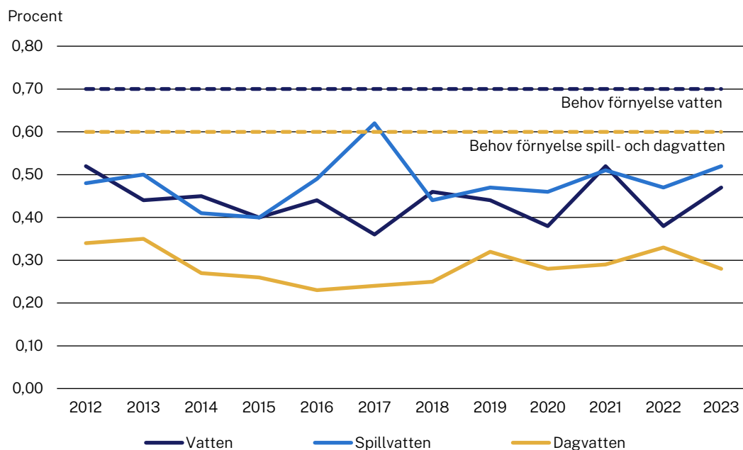
Diagram 1 Faktisk förnyelse och behov enligt Svenskt Vatten uppskattade behovet av förnyelse av ledningsnät, uppdelat på vatten samt spill- och dagvatten, 2012–2023
