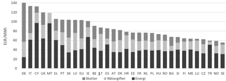
Figur 4 Industrins elpriser 2017
