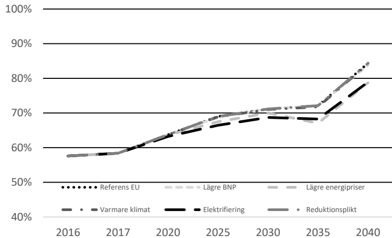
Figur 2 Scenarier till 2040
