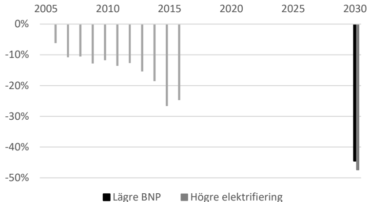
Figur 3 Scenario till 2030
