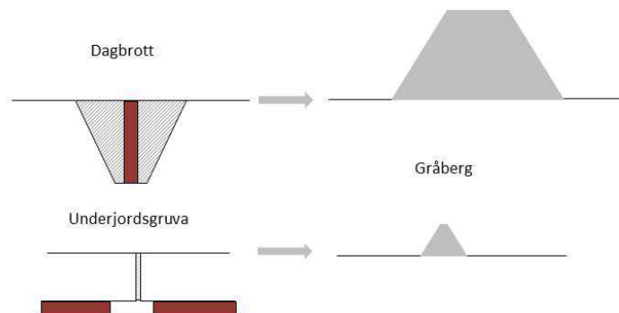
Figur 15. Gråberg vid dagbrott respektive underjordsbrytning där fiktiv malmkropp är rödmarkerad. Brytning i dagbrott innebär generellt stora mängder gråberg behöver lösgöras för att komma åt en malmkropp. Dock är mängden gråberg beroende av malmkroppens läge och utbredning. Brytning under jord innebär generellt att mindre mängder gråberg behöver lösgöras då malmkroppen inte behöver frigöras på samma sätt som vid dagbrottsbrytning.
